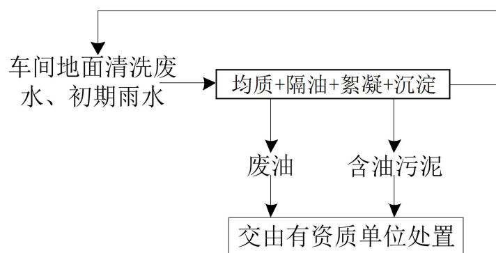
图 4-1 拟建项目污水处理站废水处理工艺流程图
