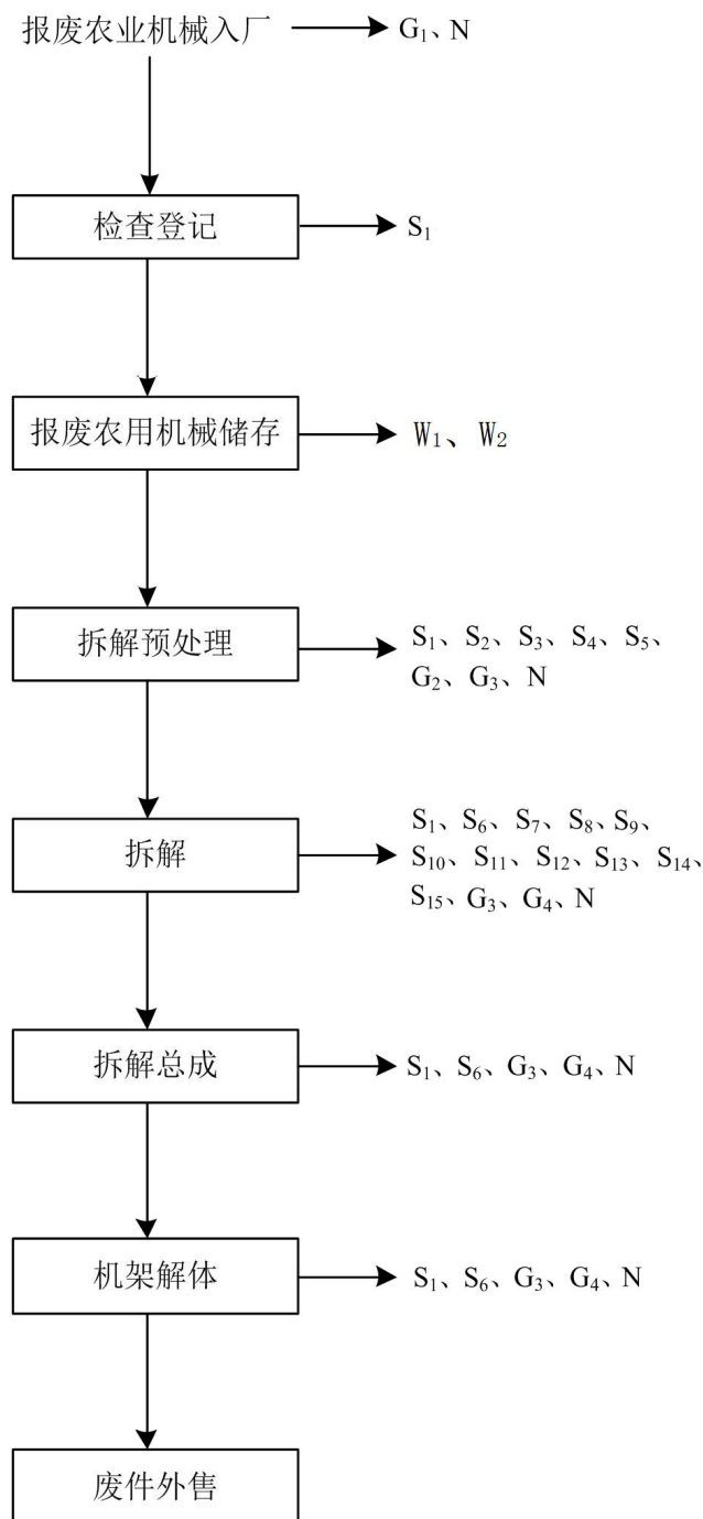
图 2-2 农机拆解生产工艺流程及产污环节图
