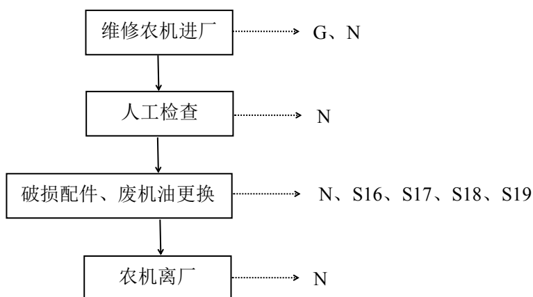
图 2-3 农机维修工艺流程及产污环节图
