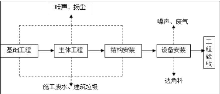
图 2-4 施工期工艺流程及产污环节图
