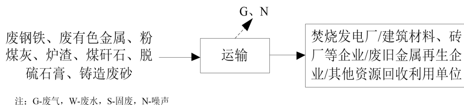
图 2-6 转运线生产工艺流程及产污环节图
