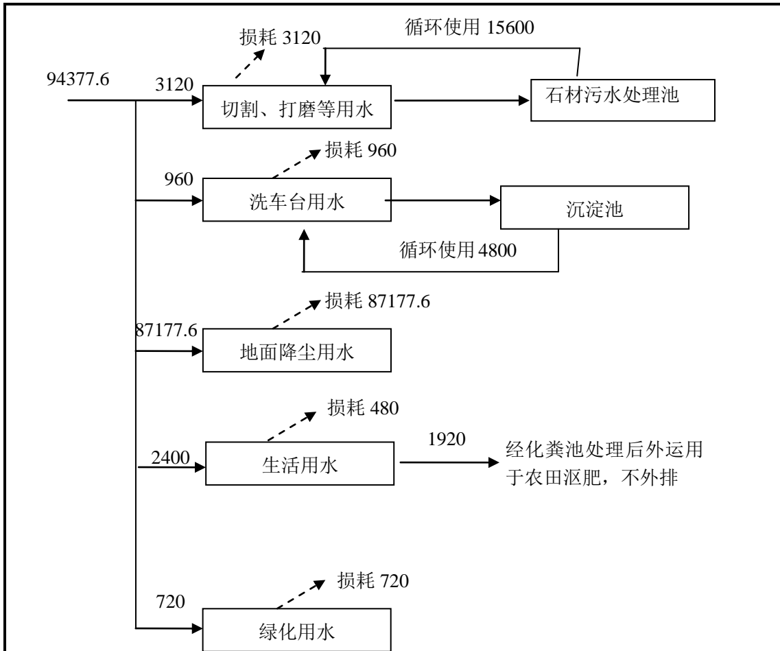
图 1-1 项目水平衡图单位: m^3/a
